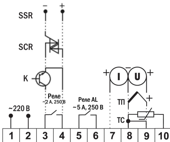
Схема подключения D49, D94, D99
